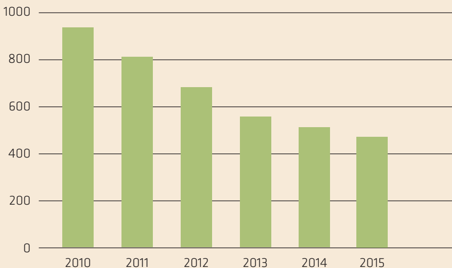
Figur 2 Den faktiske og forventede udvikling på prisen på lithium-ion batterier pr. kWh (Kilde: Pike research).
